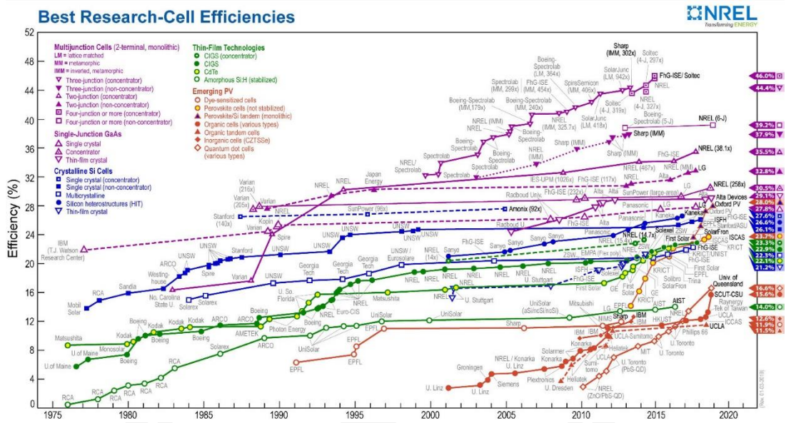
ภาพประกอบที่ 4 แผนภูมิประสิทธิภาพของโซล่าเซลล์ในชนิดต่างๆของแต่ละบริษัทหรือสถาบัน [72]
