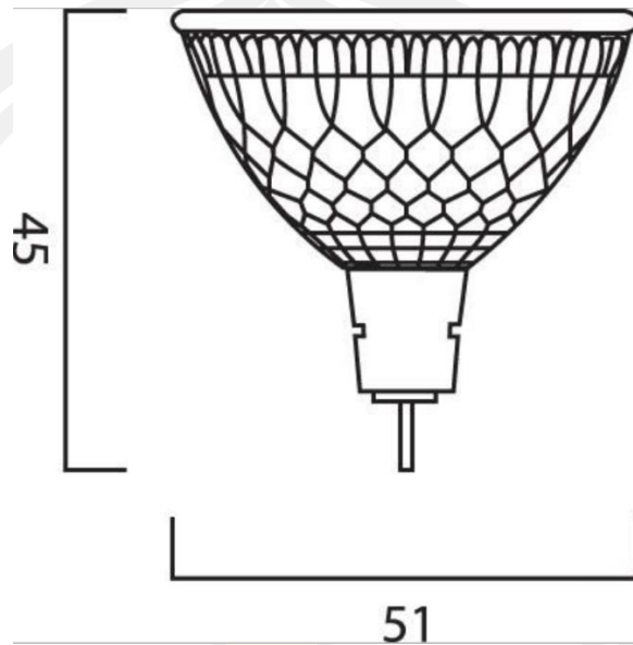
ภาพประกอบที่ 7 แสดงขนาดทางเลขาคณิตของหลอดไฟ
