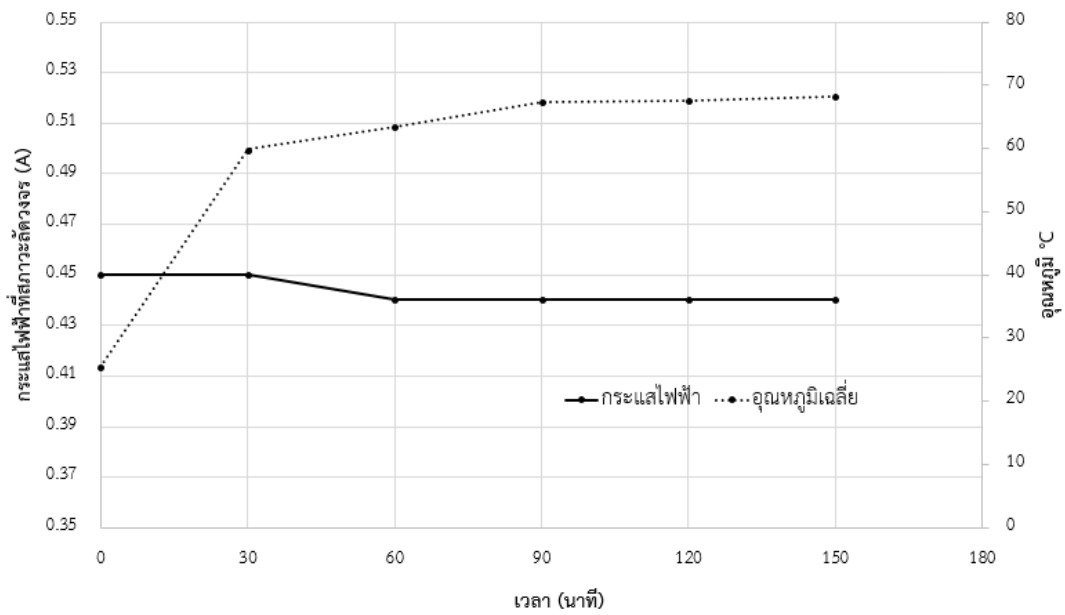
กระแสไฟฟ้าที่สภาวะลัดวงจรโดยการเชื่อมต่อแบบขนาน
