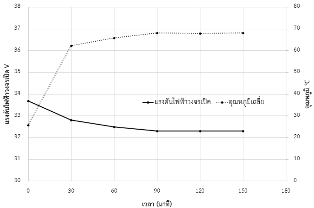
ภาพประกอบที่ 30 แสดงแรงดันไฟฟ้าวงจรถูกเปิดหลังการเชื่อมต่อโซล่าเซลล์ทั้ง 2 ชนิด แบบอนุกรม
