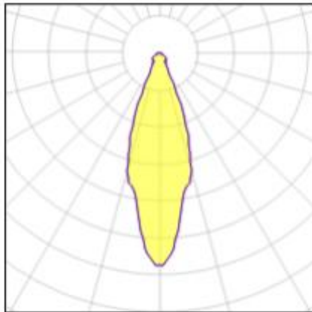
ภาพประกอบที่ 8 แสดงมุมของแสงจากหลอดไฟ
