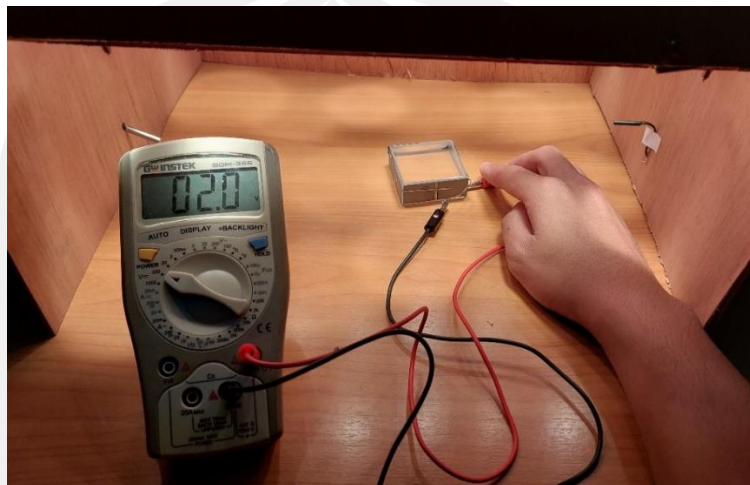
ภาพประกอบที่ 21 การทดสอบแรงดันไฟฟ้าเบื้องต้นของกริดเซลล์โปร่งแสง
