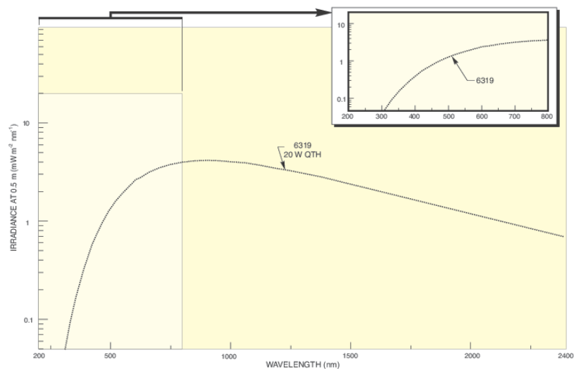
ภาพประกอบที่ 6 การปล่อยสเปกตรัมแสงของหลอดฮาโลเจน
