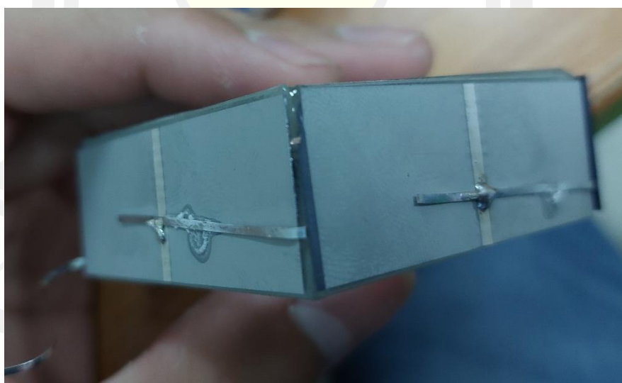
ภาพประกอบที่ 20 แสดงการเชื่อมต่อเซลล์ไฟฟ้าในกริดด้วยแทปปีงไวร์และตะกั่ว
