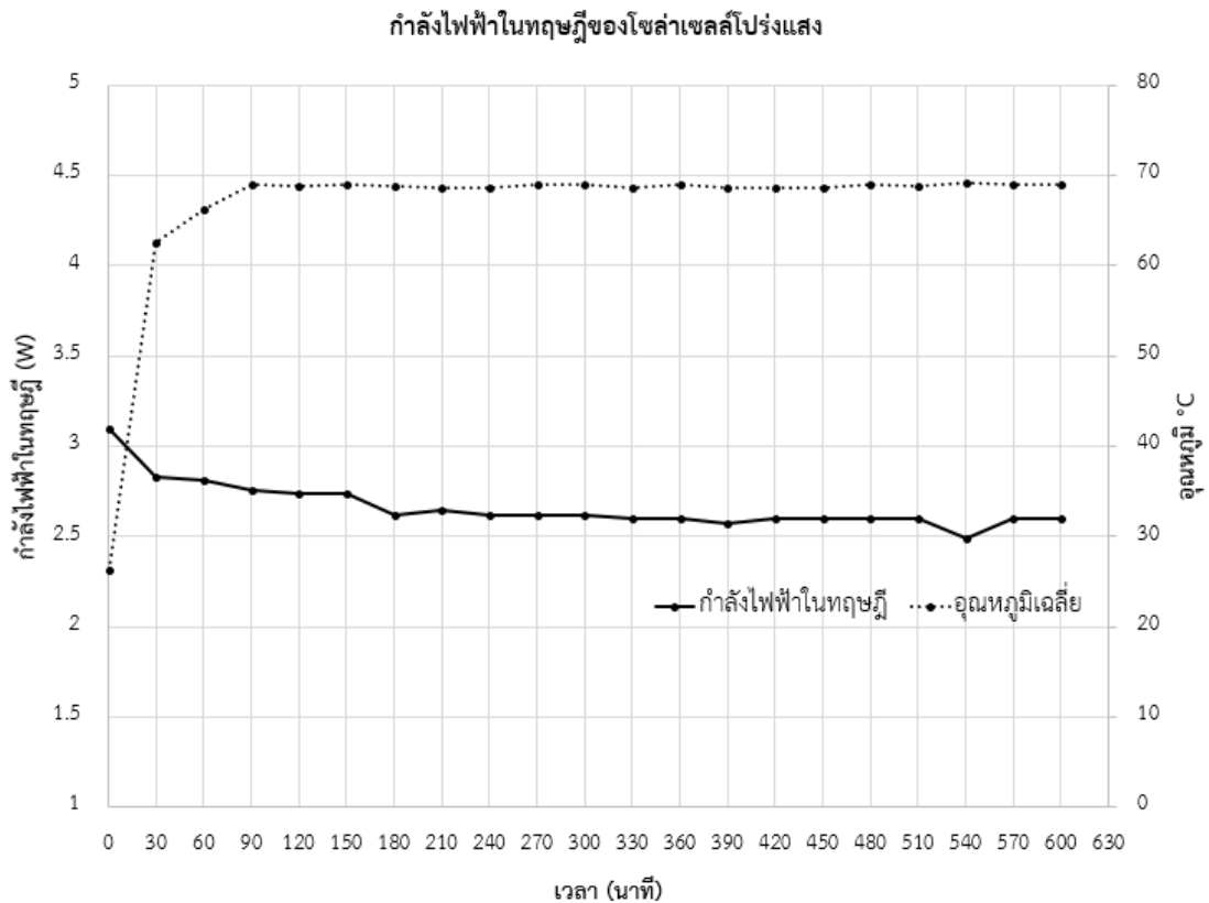
ภาพประกอบที่ 28 แสดงกำลังไฟฟ้าในทฤษฎีของโซล่าเซลล์โปร่งแสง
