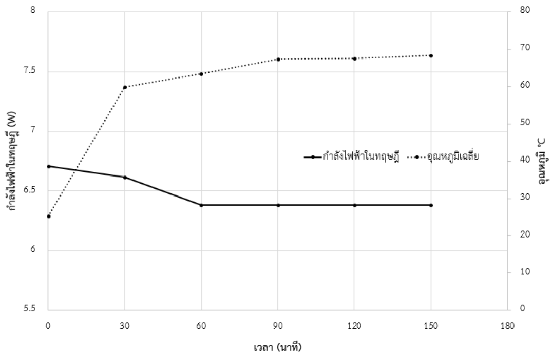
กำลังไฟฟ้าในทฤษฎีโดยการเชื่อมต่อแบบขนาน
