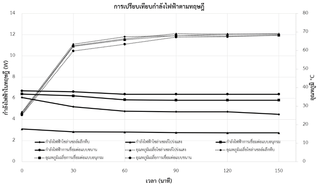
ภาพประกอบที่ 38 แสดงการเปรียบเทียบกำลังไฟฟ้าตามทฤษฎี
