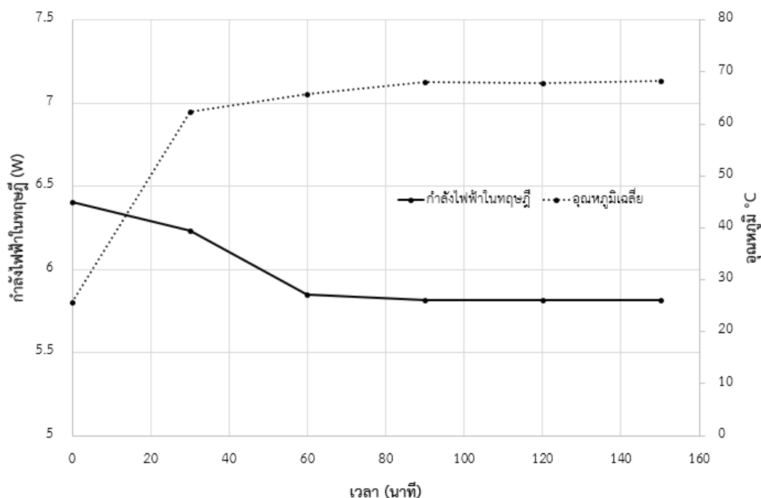
กำลังไฟฟ้าในทฤษฎีโดยการเชื่อมต่อแบบอนุกรม
