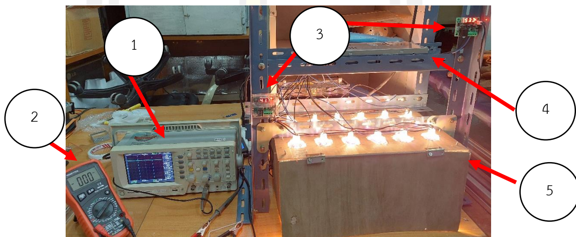
ภาพประกอบที่ 17 โครงสร้างและส่วนประกอบของห้องทดสอบระบบแสงอาทิตย์เทียม
