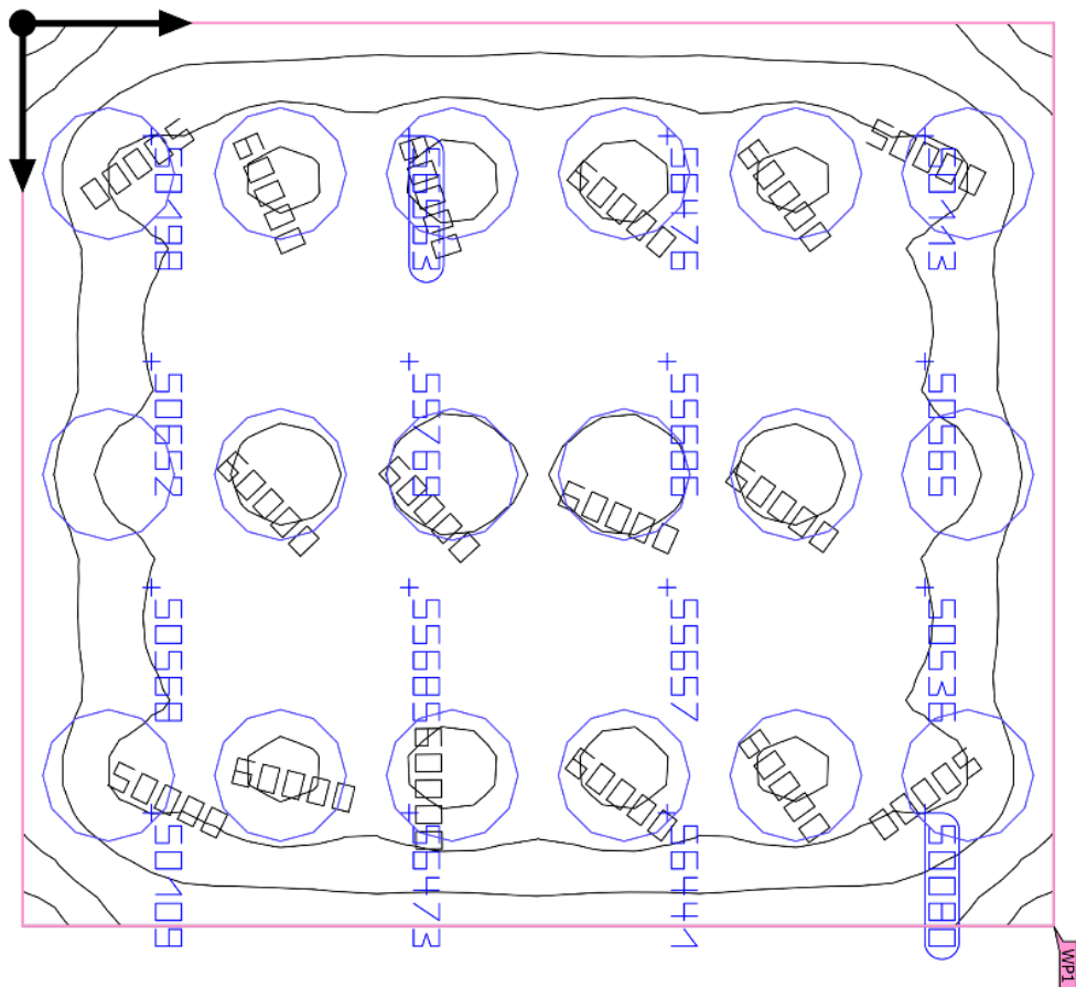
ภาพประกอบที่ 9 ผลการจำลองระบบส่องสว่างด้วยโปรแกรมไดอะลักซ์
