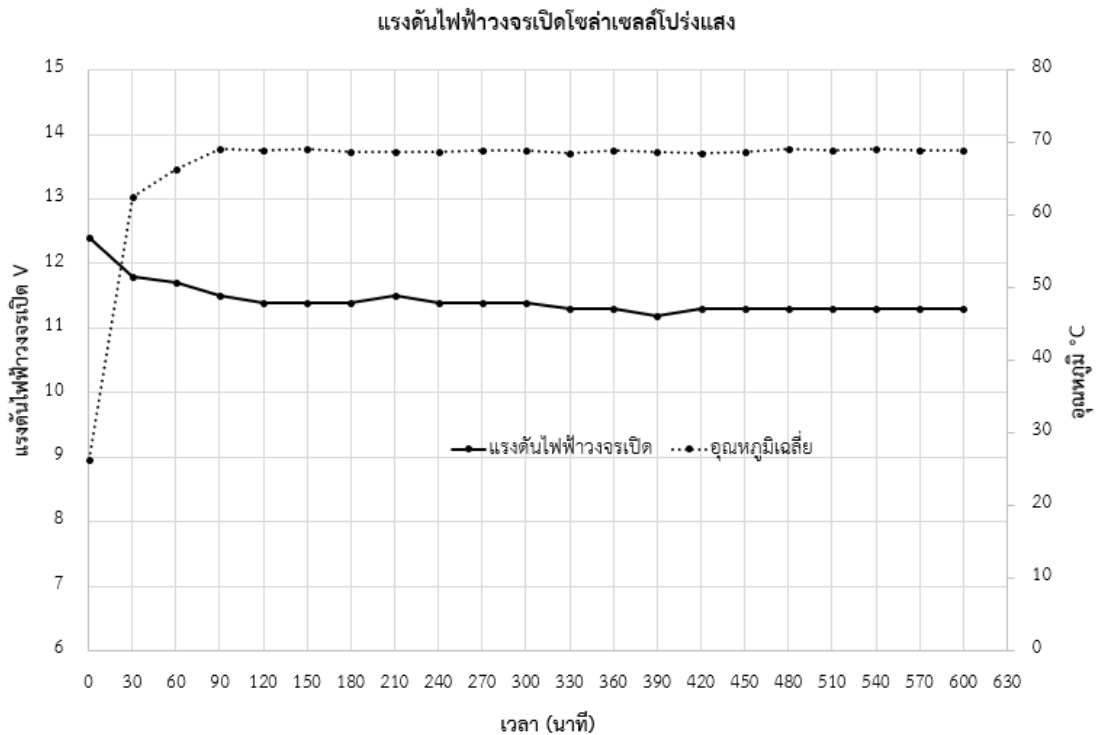
ภาพประกอบที่ 26 แสดงแรงดันไฟฟ้าวงจรถัด โซล่าเซลล์โปร่งแสง
