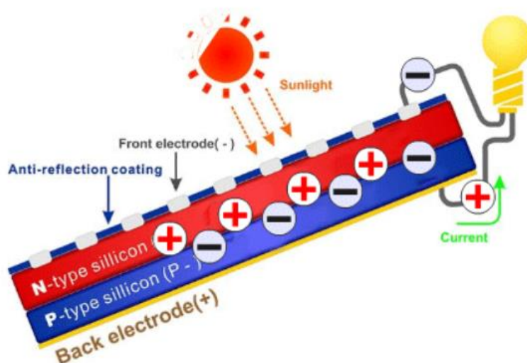
ภาพประกอบที่ 2 หลักการทำงานของโซลาร์เซลล์ [36]
