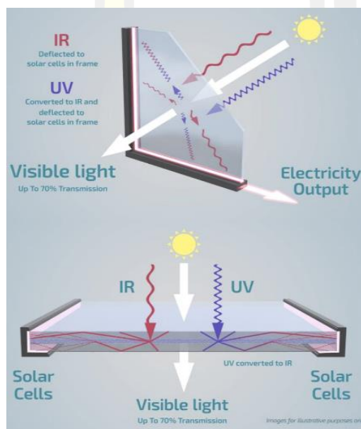
ภาพประกอบที่ 3 หลักการทำงานของโซล่าเซลล์โปร่งแสง(TLSCs) [22]
