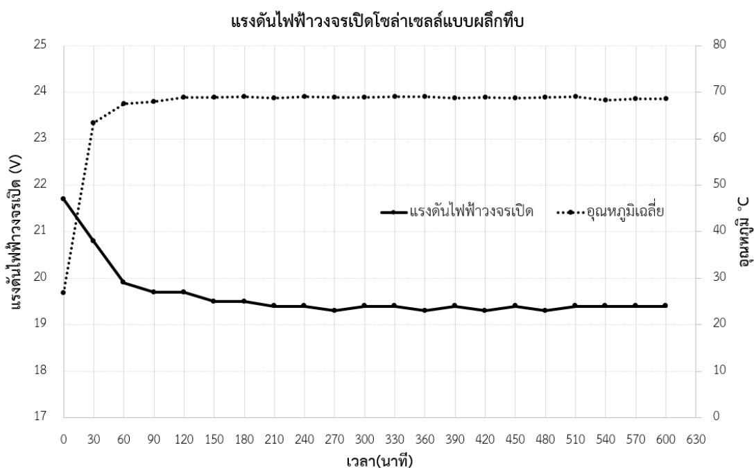
ภาพประกอบที่ 23 แรงดันไฟฟ้าวงจรเปิดของโซล่าเซลล์ผลึกทึบ
