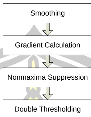
ภาพที่ 21 แสดงขั้นตอน Canny Edge Detection ที่มา [21]
