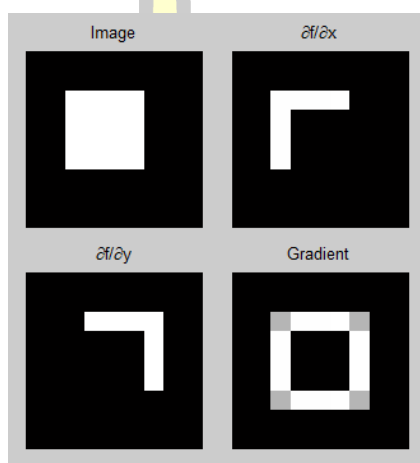
ภาพที่18 ผลการหาขอบภาพด้วยมาสก์ของโรเบิร์ตครอส
