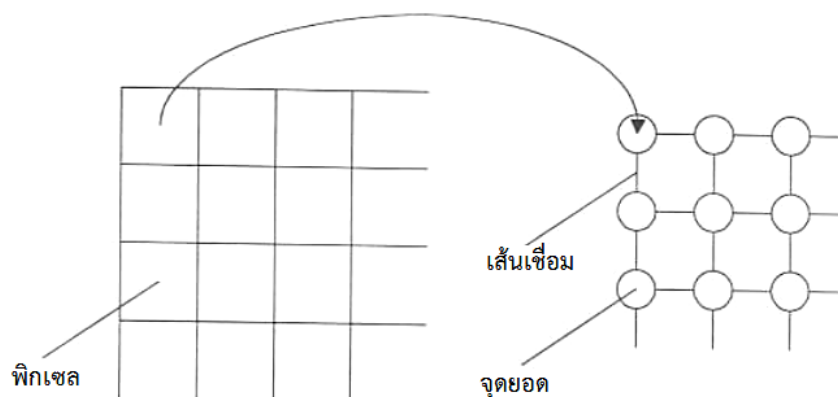
ภาพที่51 การจัดข้อมูลภาพให้อยู่ในลักษณะกราฟ ที่มา [61]
