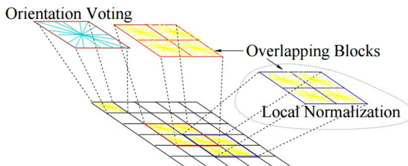
ภาพที่ 65 แสดงการซ้อนทับกันของบล็อก
