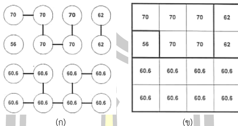
ภาพที่53 แสดงการตัดเส้นเชื่อมของข้อทดสอบแพนนิ่งทรี ที่มา [64]
