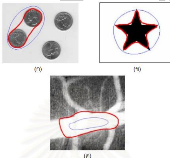
ภาพที่ 48 ปัญหาของการแบ่งส่วนภาพโดยใช้ Active Contour ตามวิธีการของ Kass ที่มา [50]
