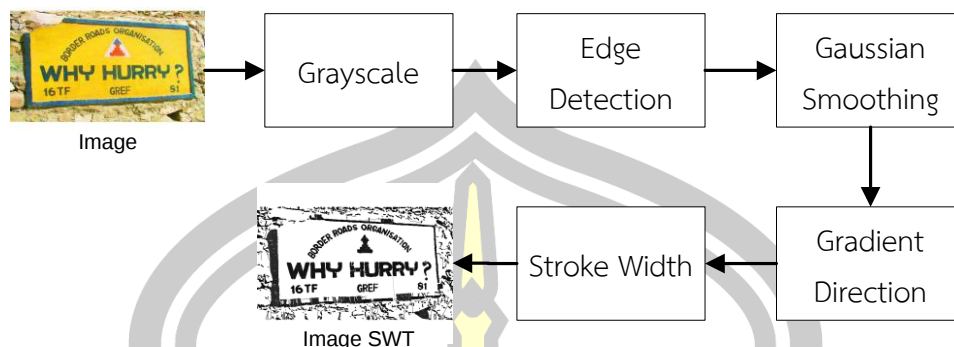
ภาพที่ 37 กระบวนการ The Stroke Width Transform
