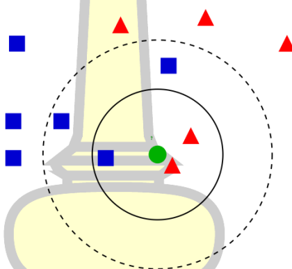
ภาพที่ 5 แสดงการจำแนกประเภทด้วยวิธีเพื่อนบ้านใกล้ที่สุด
