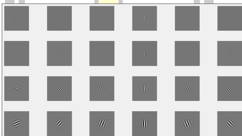
ภาพที่ 36 รูปร่างที่เป็นองค์ประกอบส่วนจินตภาพของตัวกรองกาบอร์
