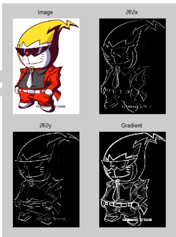
ภาพที่20 ผลการหาขอบภาพด้วยวิธีโซเบล
