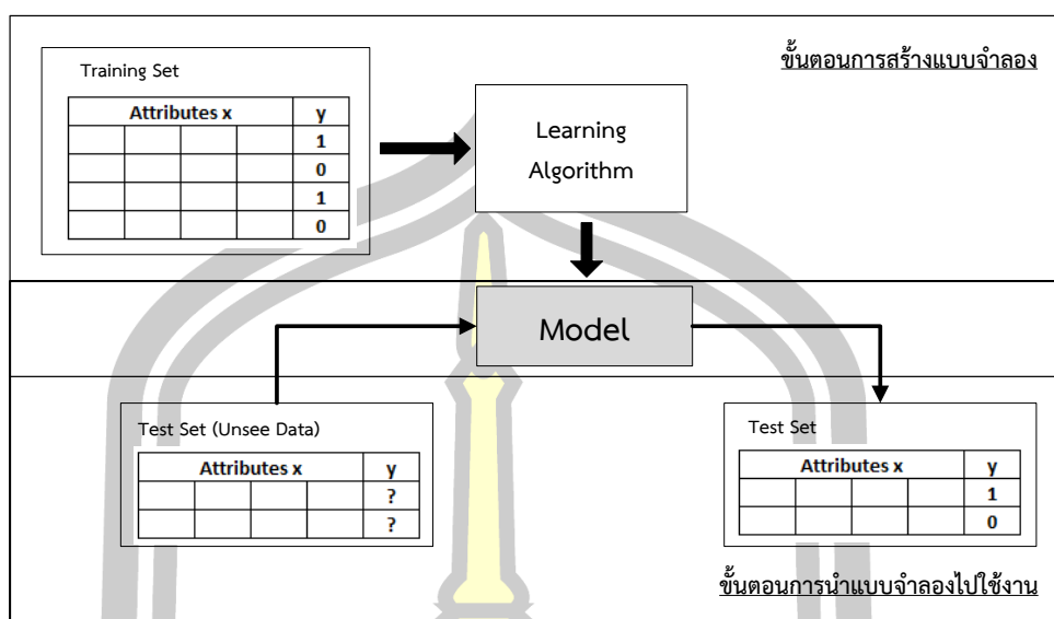
ภาพที่ 67 ขั้นตอนของการจำแนกประเภท ที่มา [73]
