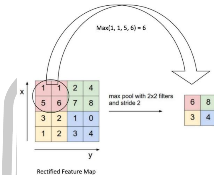
ภาพที่ 73 การพูลลิงค่ามากที่สุด
