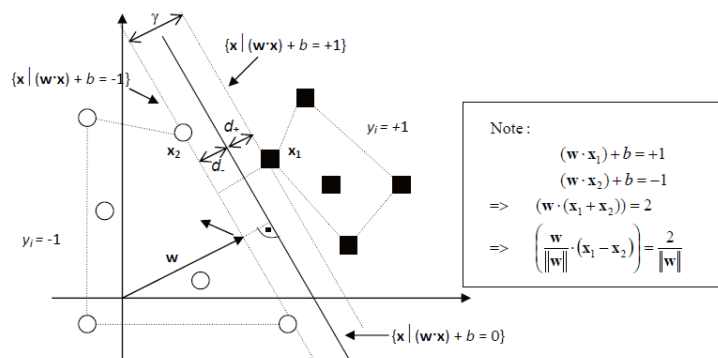
ภาพที่ 6 การแบ่งกลุ่มข้อมูลตัวอย่างด้วยไฮเปอร์เพลนโดยใช้เทคนิค SVM ที่มา [9]
