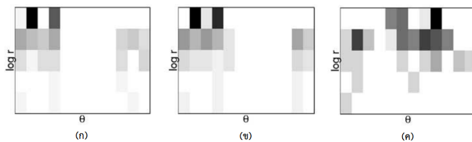
ภาพที่ 57 (ก) ค่า Shape Context ของอักษร A ณ จุดอ้างอิง X1 (ข) ค่า Shape Context ณ จุดอ้างอิง X2 และ (ค) ค่า Shape Context ณ จุดอ้างอิง X3 ที่มา [66]
