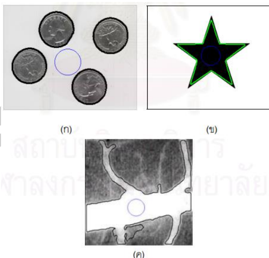
ภาพที่ 49 การแบ่งส่วนภาพโดยวิธีการเลเวลเซต ที่มา [50]
