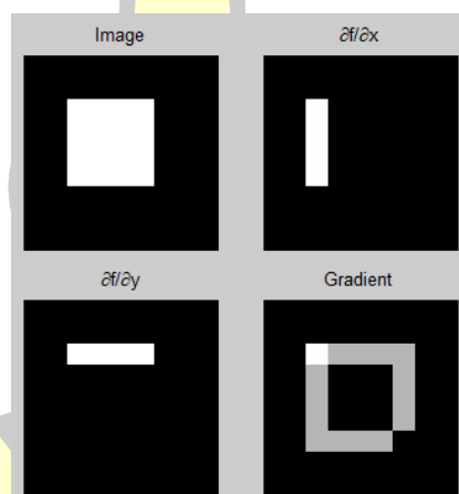
ภาพที่17 ผลการใช้มาสก์อย่างง่ายเพื่อหาขอบของวัตถุสี่เหลี่ยมสีขาวขนาด 4x4 พิกเซล บนพื้นสีดำขนาด 9x9 พิกเซล
