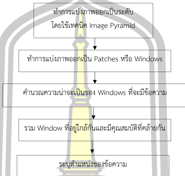
ภาพที่132 แสดงภาพรวมของเทคนิคในการตรวจจับข้อความในภาพโดยใช้ข้อมูลก่อนหน้า (Prior Information)
