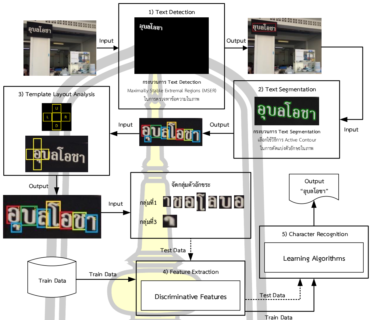
ภาพที่120 กระบวนการตรวจจับและการรู้จำอักขระ
