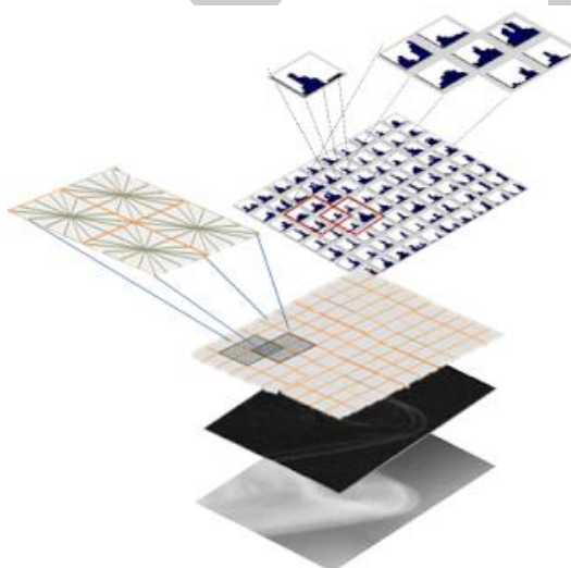
ภาพที่ 62 แสดงกระบวนการสกัดคุณลักษณะของ HOG
