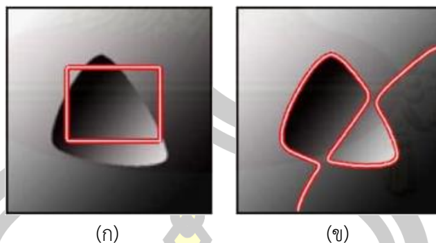
ภาพที่44 การแบ่งส่วนภาพในกรณีที่ทั้งวัตถุและพื้นหลังเป็นเนื้อผสมโดย (ก) คอนทัวร์เริ่มต้น (ข) ผลการแบ่งส่วนภาพที่ได้ ที่มา [37]
