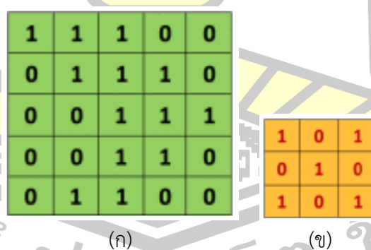
ภาพที่ 69 จำลองเมทริกซ์ที่ได้จากรูปที่รับเข้ามาและเมทริกซ์ตัวกรองค่า
