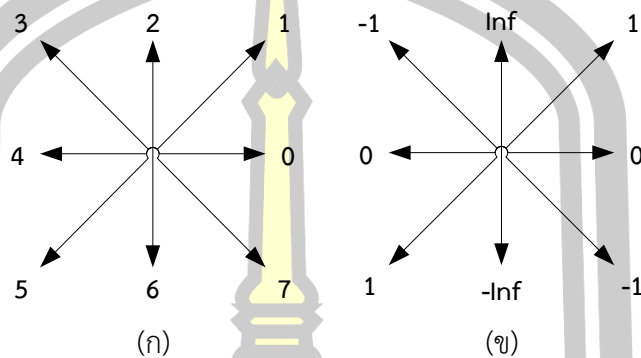
ภาพที่117 (ก) ค่าทิศทางของ Freeman Chain Code แบบเดิม (ข) ค่าทิศทางของ Freeman Chain Code แบบใหม่
