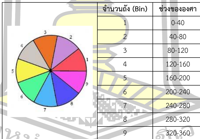
ภาพที่ 161 แสดงการกำหนดถังกับทิศทาง 0-360 องศา
