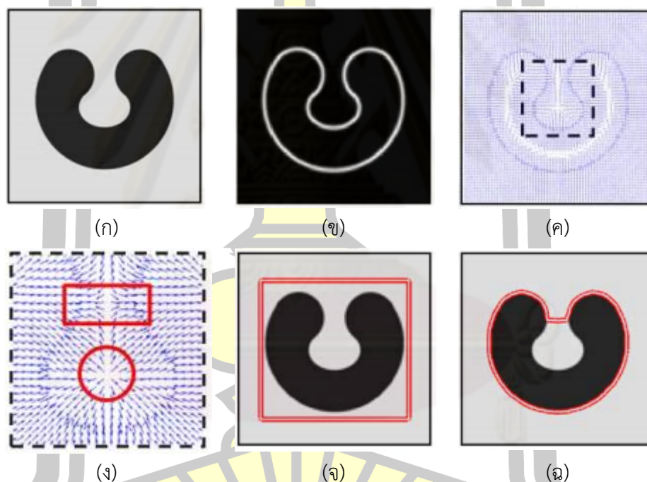
ภาพที่ 4.2 ปัญหาจุดอานม้าและจุดหยุดนิ่ง (ก) ภาพรูปตัวยูที่บริเวณตรงกลางมีลักษณะคล้ายอ่าว (ข) ภาพขอบ (ค) ภาพสนามเวกเตอร์ที่ได้ (ง) จุดอานม้า (แสดงในสี่เหลี่ยม) และจุดหยุดนิ่ง (แสดงในวงกลม) (จ) คอนทัวร์เริ่มต้น (ฉ) ผลการแบ่งส่วนภาพที่ได้ ที่มา [37]
